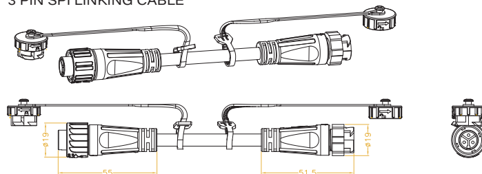
3 PIN SPI LINKING CABLE
