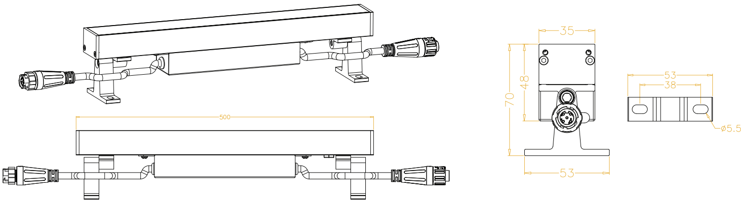
BXG40 DIMENSIONS – 500MM
