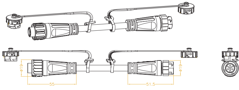
3 PIN SPI LINKING CABLE
