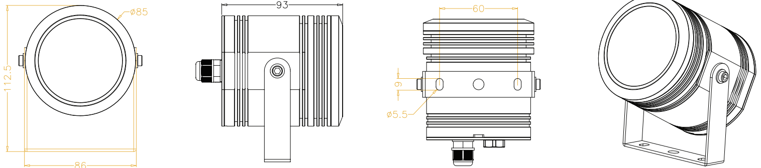
BXS10 DIMENSIONS – NO SNOOT
