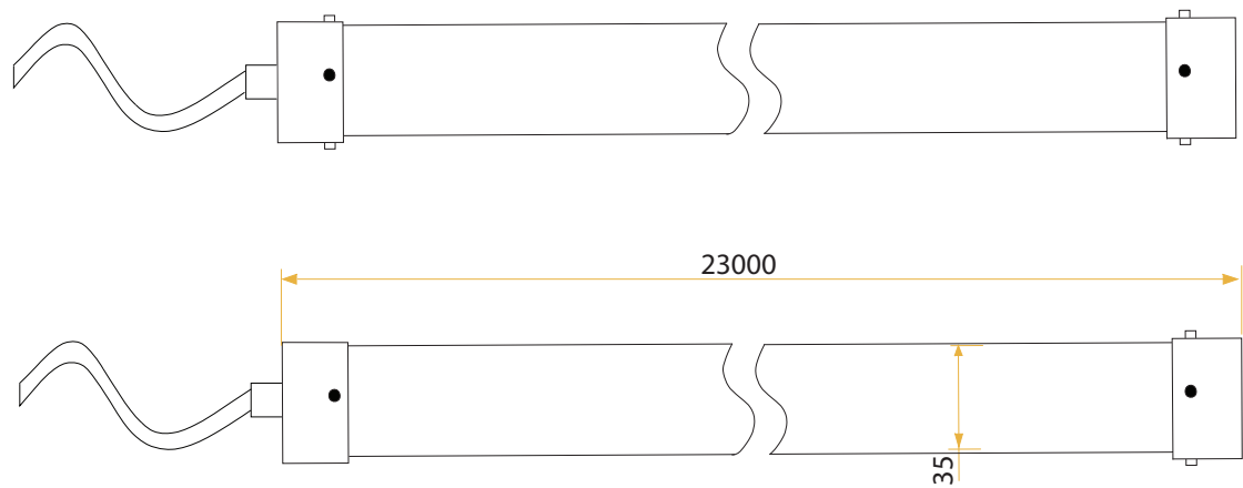
RXN35 DIMENSIONS
