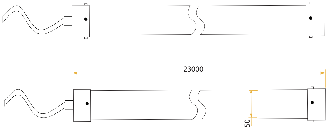
RXN50 DIMENSIONS
