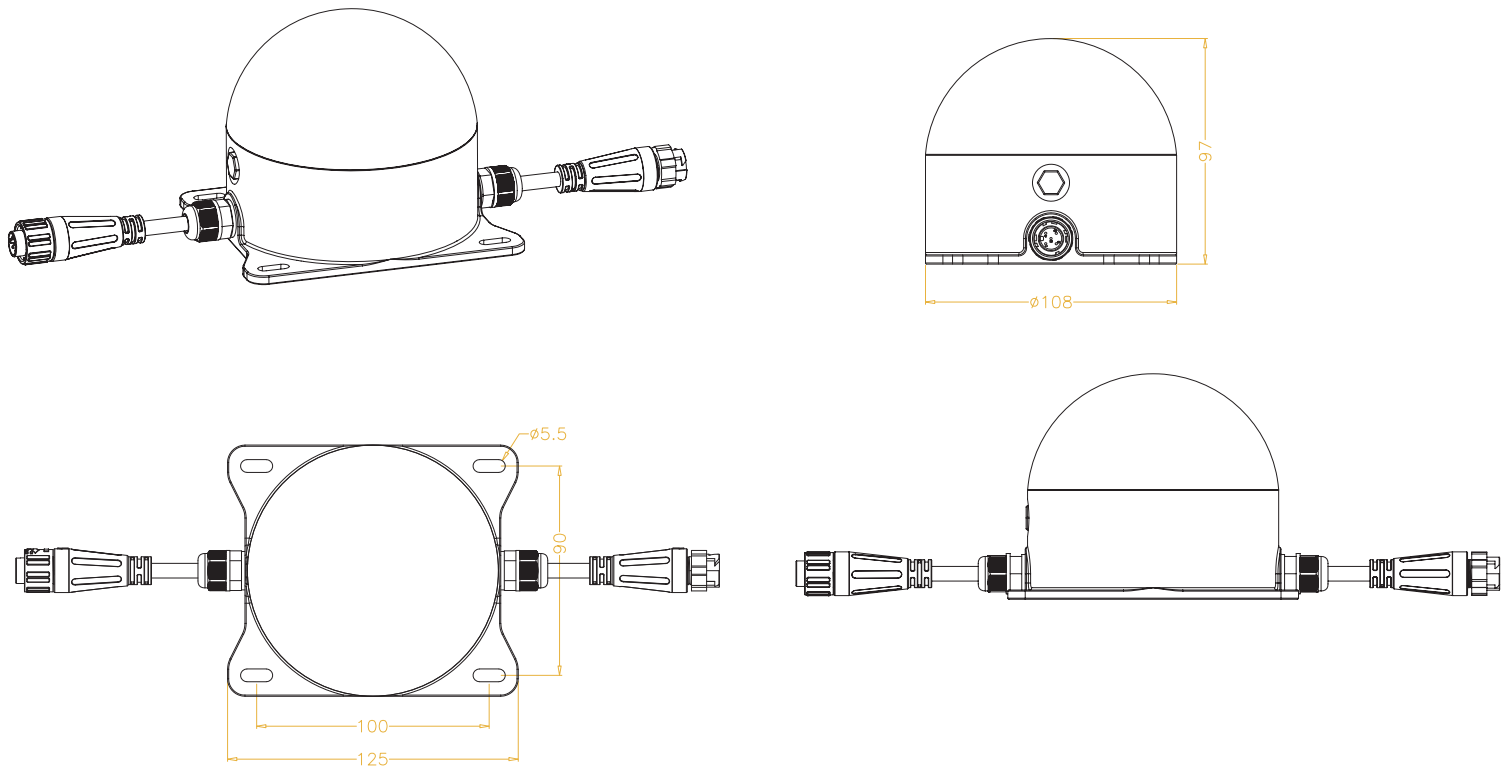
XAD 14 DIMENSIONS
